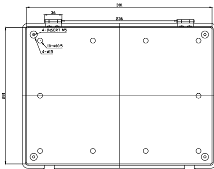
BODY-BOTTOM
