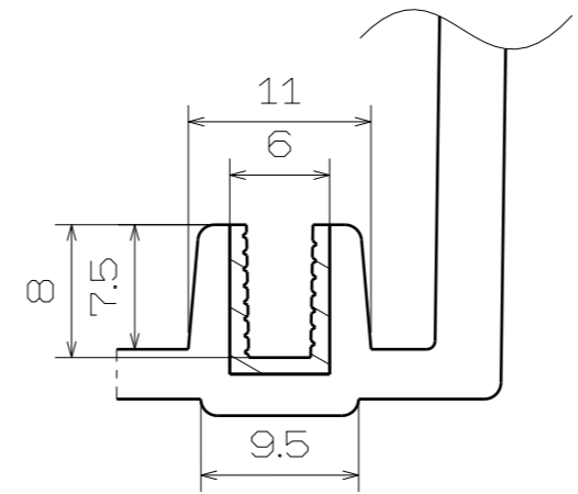
切断図F-F スケール 2:1
