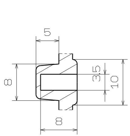
断面図E-E スケール 2:1
