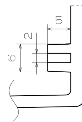
断面E-E スケール 2:1
