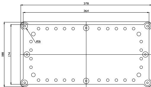
BODY-BOTTOM
