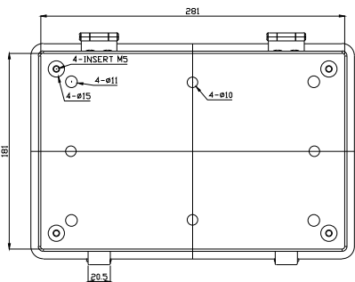
BODY-BOTTOM
