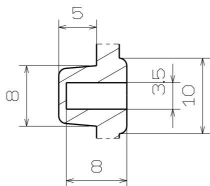
断面図 F-F スケール: 2:1
