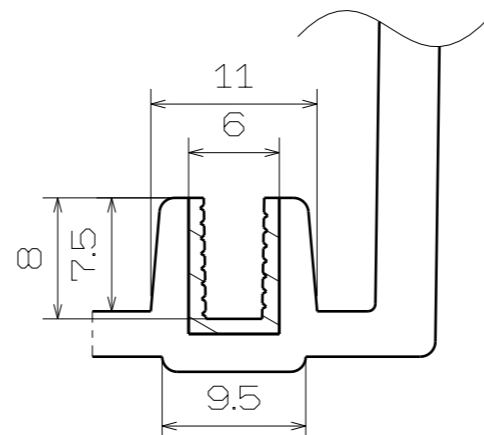
切断図 F-F スケール: 2:1
