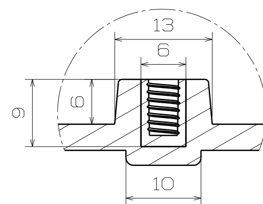
部分放大图 D 对图 21
