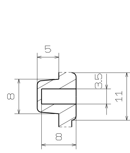
断面図-F スケール 2:1
