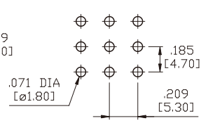
3P
