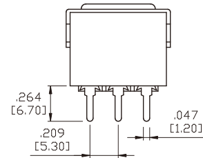
3P
