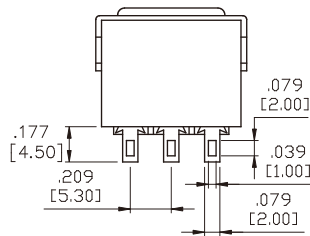
3P
