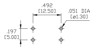
P.C.B LAND PATTERN
