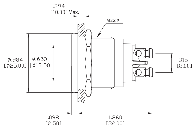
T-Flat bezel
