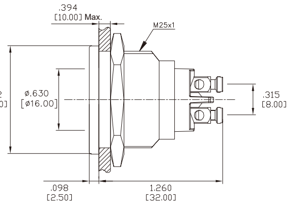
T-Flat bezel
