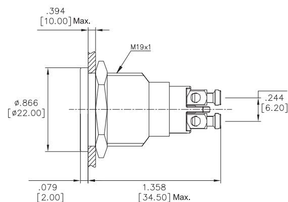
T-Flat bezel
