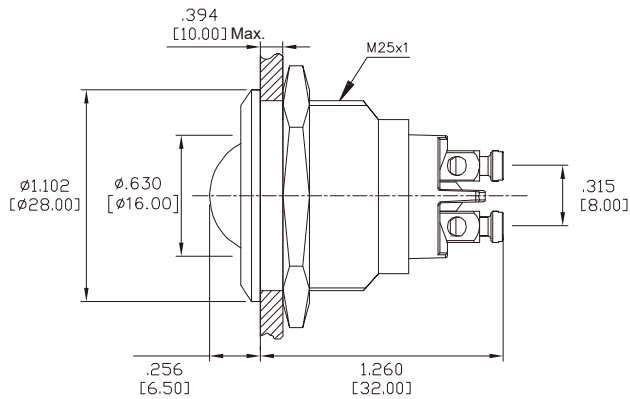
Domed bezel
